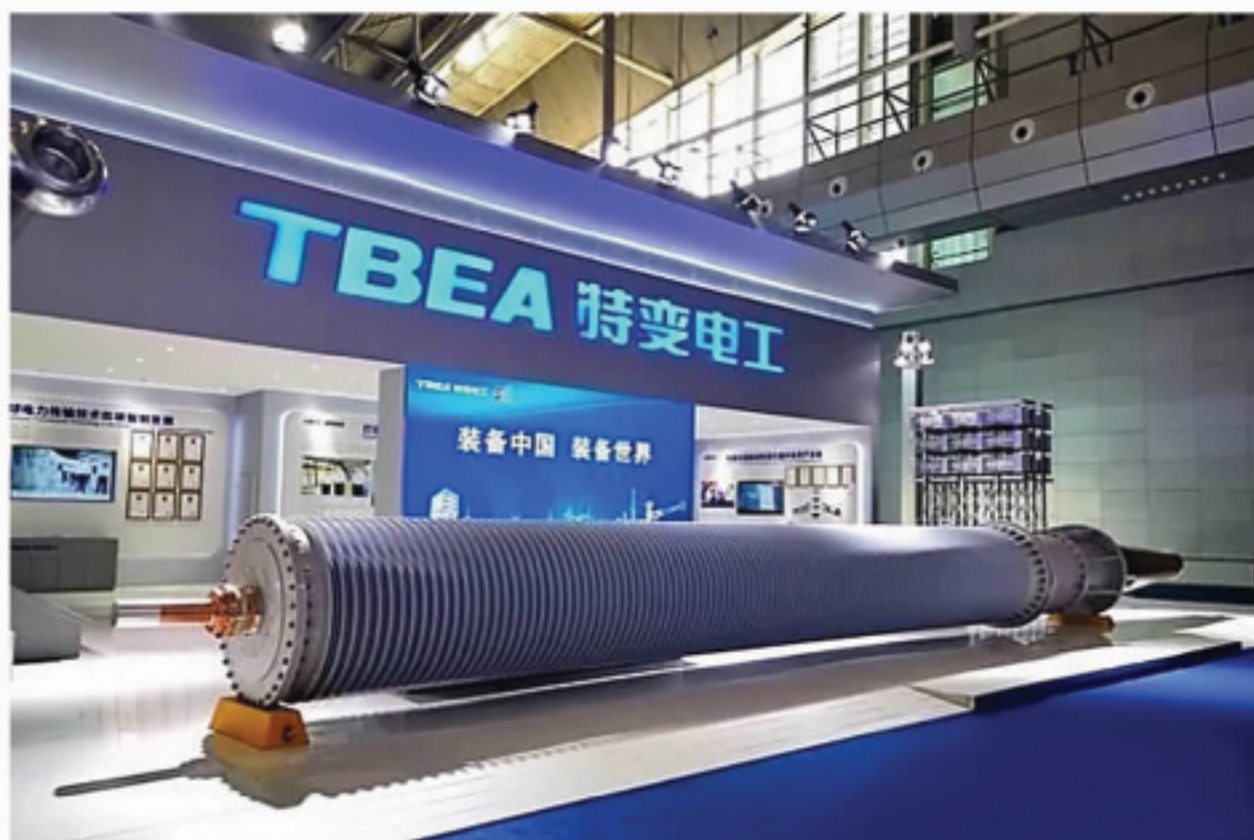
第七届中国—亚欧博览会（特变电工）国内首支 \pm 800 千伏特高压干式直流套管
